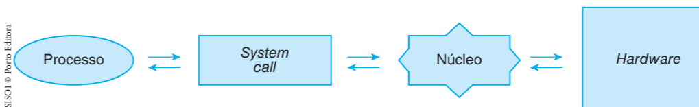
Fig. 1.5 Chamada ao sistema (system call)
