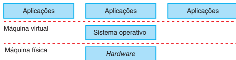
Fig. 1.2 Sistema operativo
