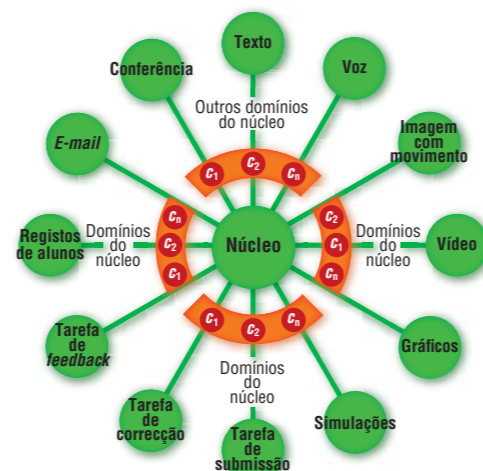
Fig. 1.3 Núcleo (kernel)
